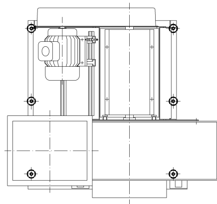
Kilremsdrift
