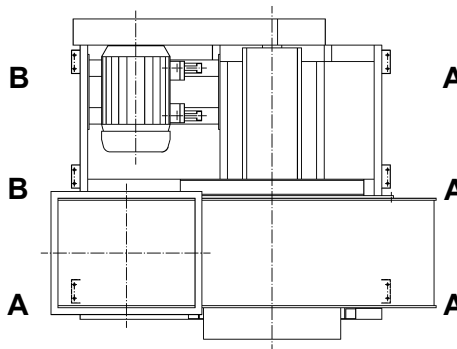
Kilremsdrift
