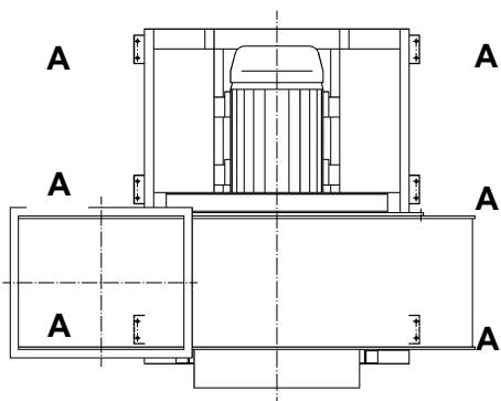
Direktdrift
