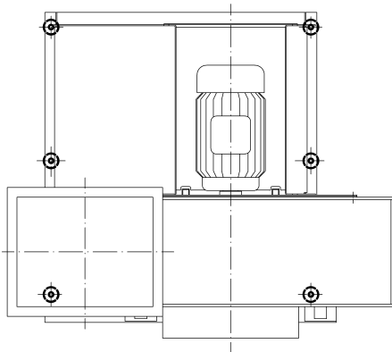
Direktdrift
