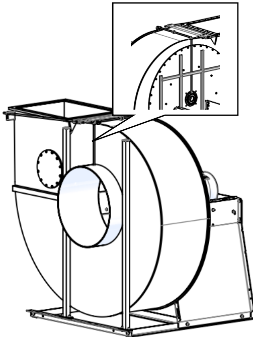
Alternativ Baksugning
