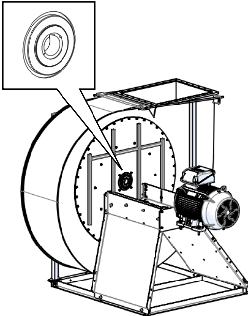
Läpptätningar enkelt
