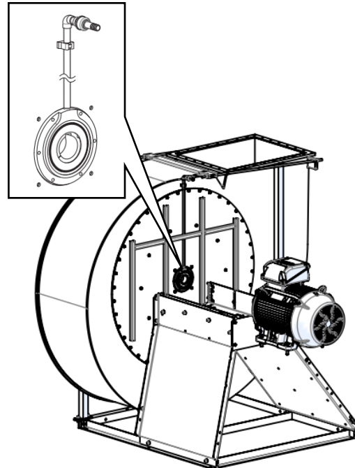
Alternativ Spärrgas
