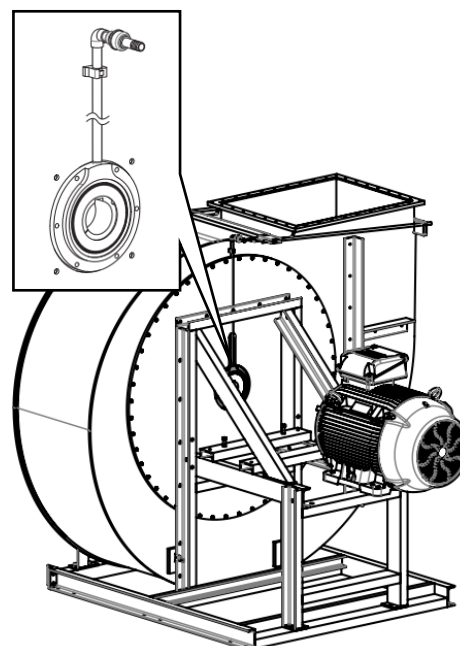
Alternativ Spärrgas
