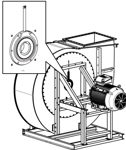
Dubbel tätning med smörjnipplar
