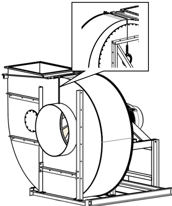
Alternativ Baksugning
