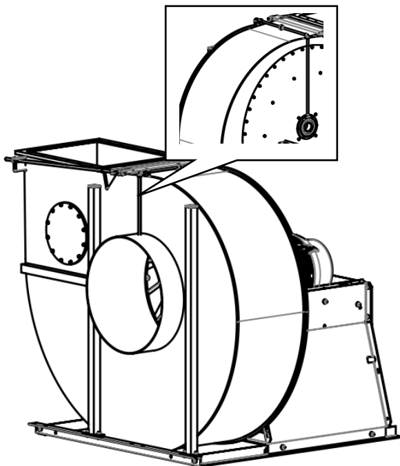
Alternativ Baksugning
