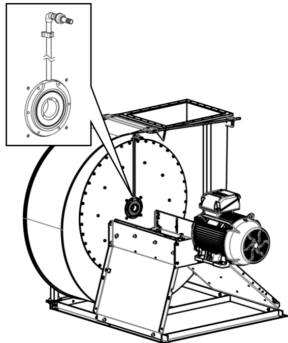
Alternativ Spärrgas
