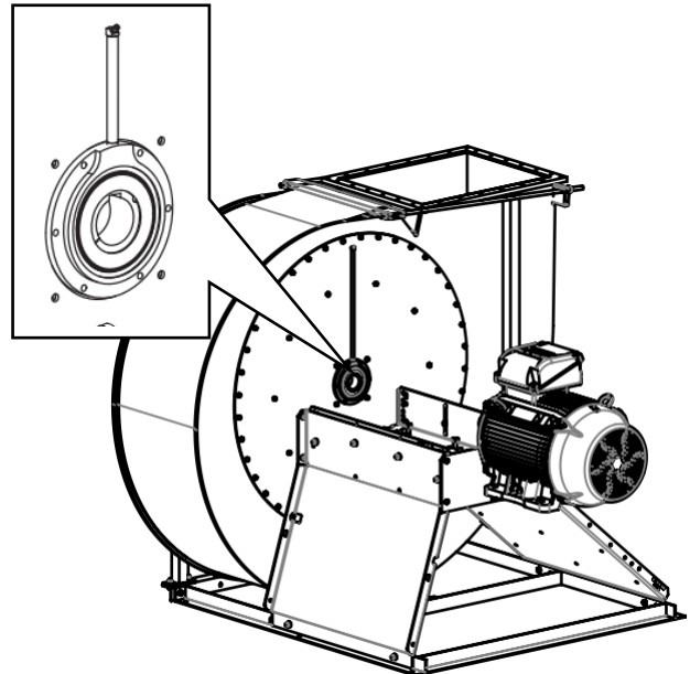
Dubbel tätning med smörjnipllar
