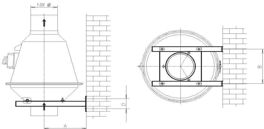
Bild 17: Monteringsmassa
