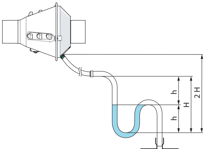
Bild 24: Sifon- och monteringshöjd
