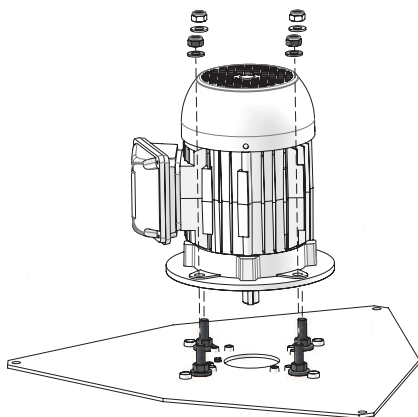
Bild 31: Demontera elmotor
