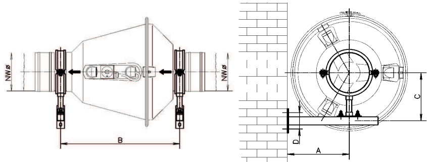
Bild 15: Monteringsmassa
