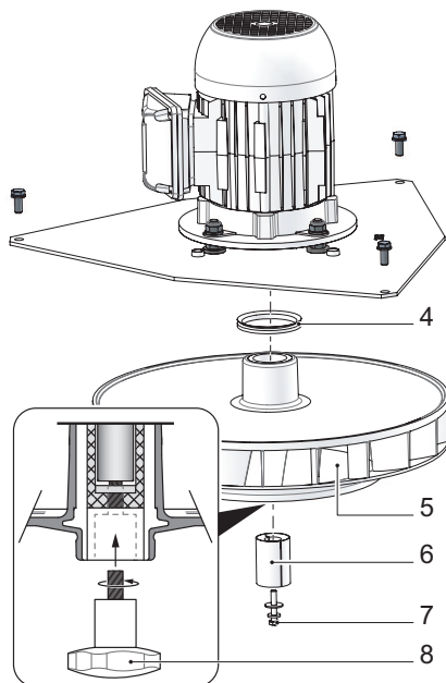
Bild 30: Demontera fläkthjul
