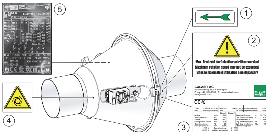
Bild 3: Skyltar och varningssymboler på fläkten
