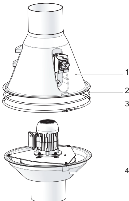
Bild 28: Demontera hus
