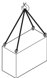
Bild 18: Kolli med öglebultar
