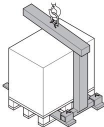
Bild 19: Kolli på transportpall
