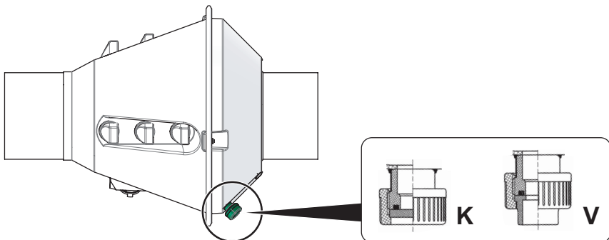
Bild 23: Kondensatstosens korrekta position
