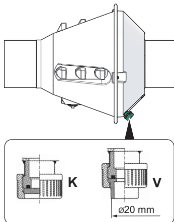
Bild 7: Kondensatstos på kondensatutlopp
