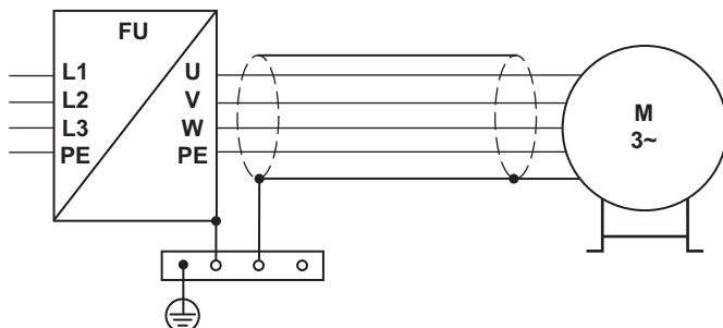
Bild 25: Anslutningsprincip för kort motorkabel (FO nära fläkten)
