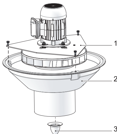
Bild 29: Avlägsna navskyddet och motorplattan
