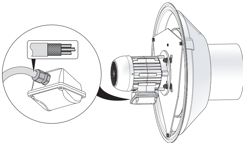
Bild 26: EMC-kabelförskruvning
