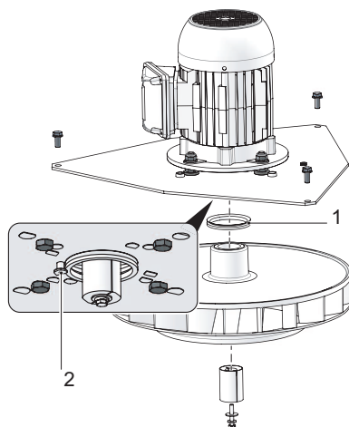
Bild 33: Ersätt V-ring-tätning
