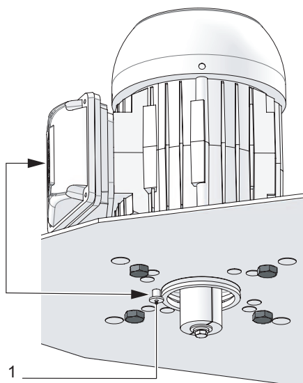
Bild 32: Placera elmotorn
