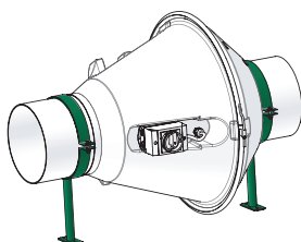
Bild 12: Golv- eller takmontering
