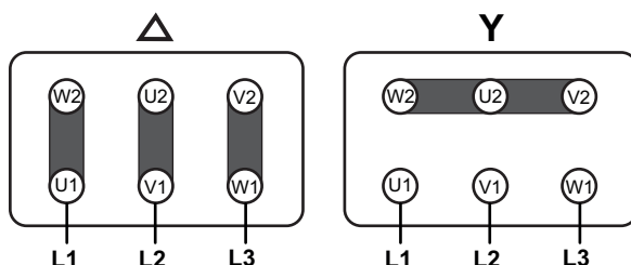
Bild 27: Anslutningskonfiguration för D- och stjärnkoppling
