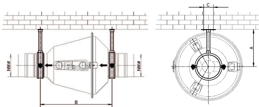
Bild 13: Monteringsmassa
