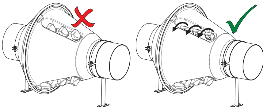
Bild 21: Rikta luftstosen horisontellt vid uppställning utomhus
