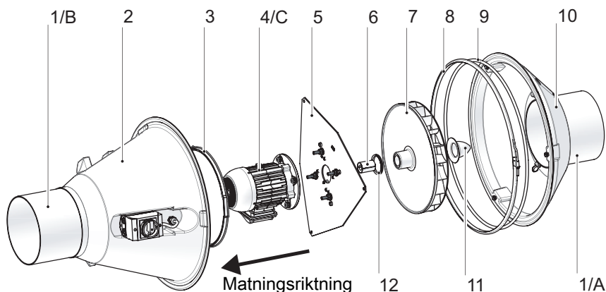
Bild 2: Fläkt-översikt
