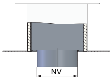
b) Röranslutning
