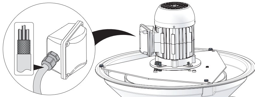
Bild 16: EMC-kabelförskruvning
