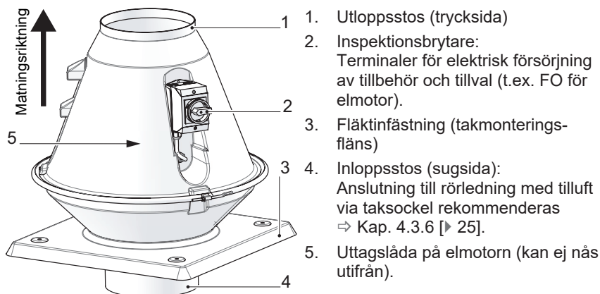
Bild 1: Gränssnitt på fläkten
