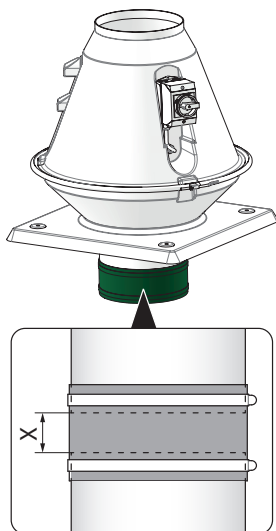
Bild 13: Röranslutningarnas distansområde
