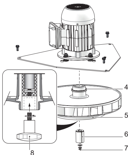
Bild 20: Demontera fläkthjul
