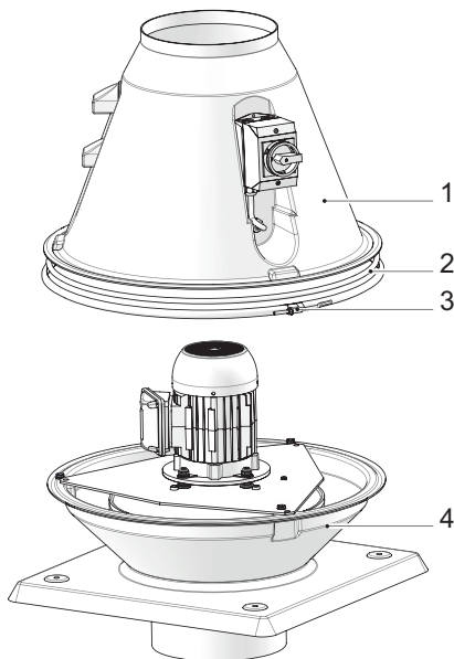
Bild 18: Demontera hus
