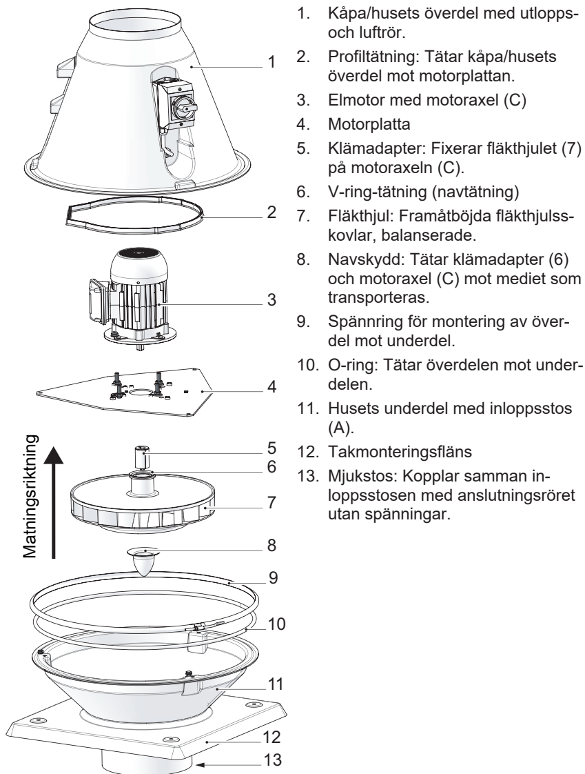
Bild 2: Fläkt-översikt
