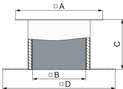
a) Avsnitt tak (rektangulär anslutning)
