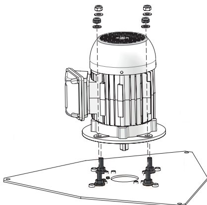
Bild 21: Demontera elmotor
