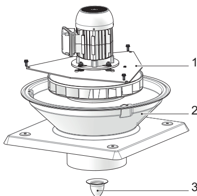
Bild 19: Avlägsna navskyddet och motorplattan
