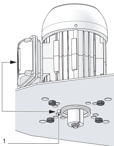
Bild 22: Placera elmotorn
