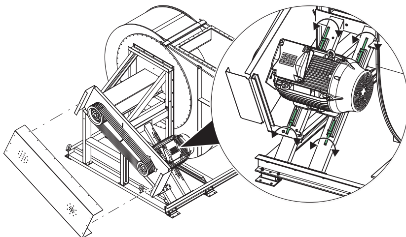
Bild 45: Ersätt drivrem
