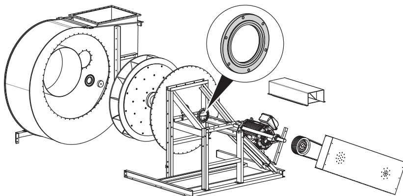
Bild 42: Ersätt läpptätning
