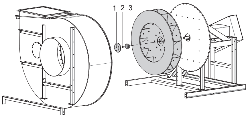
Bild 39: Byta fläkthjul
