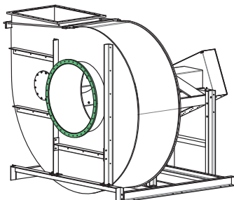
Bild 7: Rund flänsanslutning
