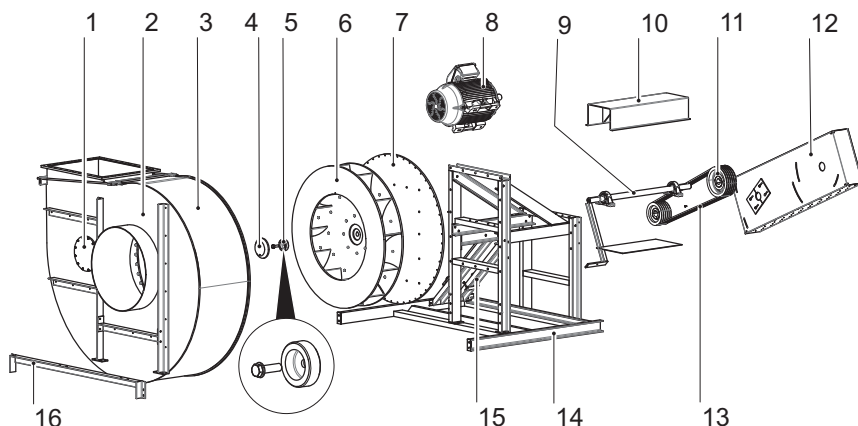
Bild 2: Fläkt-översikt
