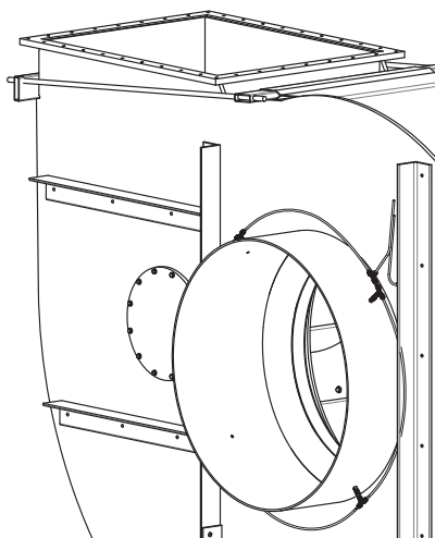
Bild 44: Byt ut huvudringen
