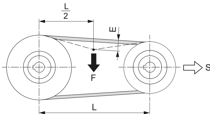
Bild 46: Mät remspänning
