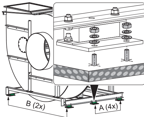
Bild 29: Fastsättningsförslag för golvmontering
