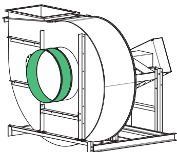
Bild 5: Mjukstosarnas monteringspositioner
