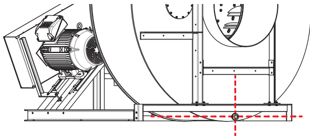
Bild 31: Kondensatstosens korrekta position
