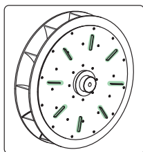
Bild 16: Labyrint-navtätning
