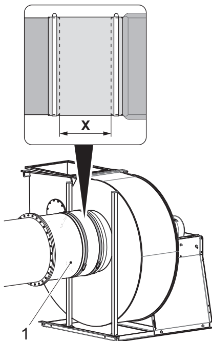
Bild 29: Röranslutningarnas distansområde
