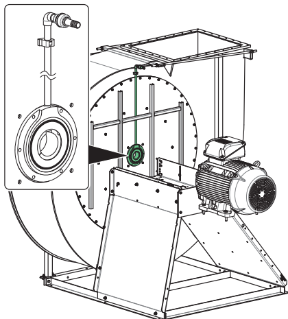
Bild 14: Spärrgasanslutning
