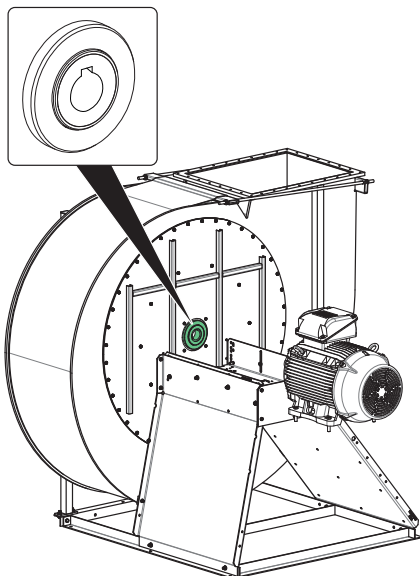
Bild 15: Filtring navtätning
