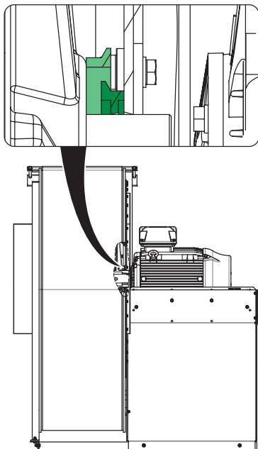
Bild 16: Labyrint-navtätning
