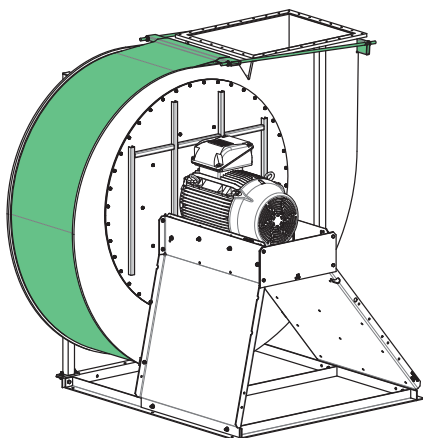
Bild 26: Korrekt montering av splitterskyddet
