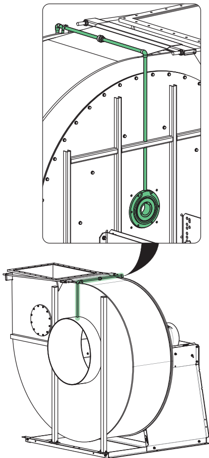
Bild 13: Baksugning
