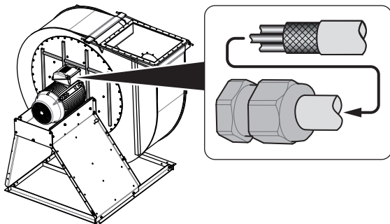
Bild 34: EMC-kabelförskruvning
