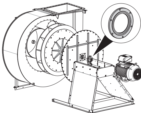
Bild 39: Ersätt läpptätning
