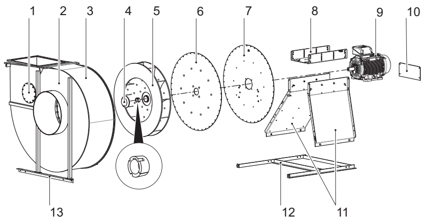
Bild 2: Fläkt-översikt
