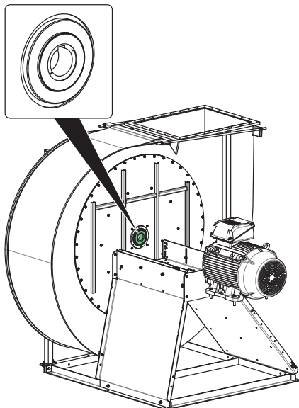
Bild 11: Läpptätning (enkel)
