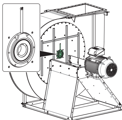
Bild 12: Dubbeltätning med eftersmörjningsnippel
