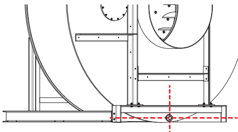
Bild 30: Kondensatstosens korrekta position
