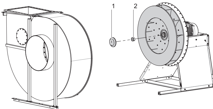
Bild 37: Byta fläkthjul
