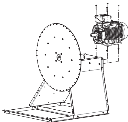
Bild 38: Demontera elmotor
