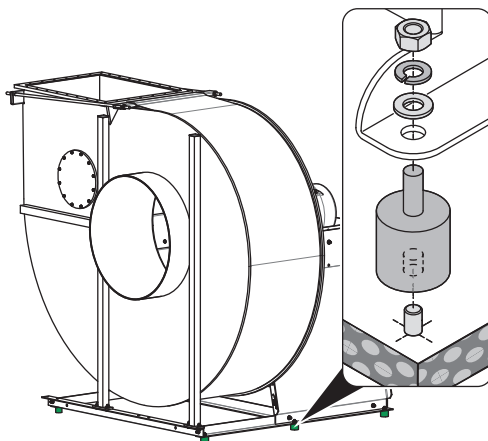
Bild 28: Fastsättningsförslag för golvmontering
