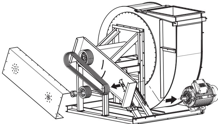
Bild 40: Demontera elmotor
