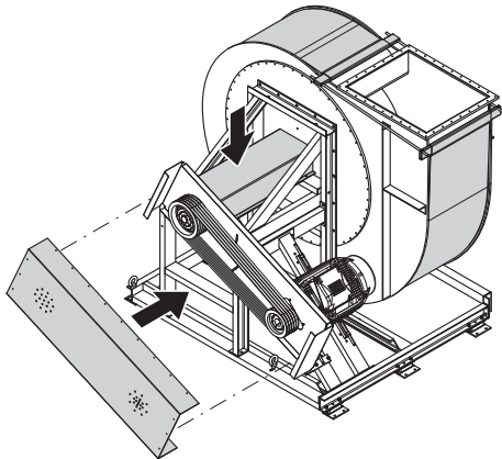
Bild 33: Kontrollera splitterskydd och skyddskåpor
