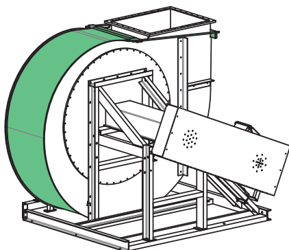
Bild 26: Korrekt montering av splitterskyddet
