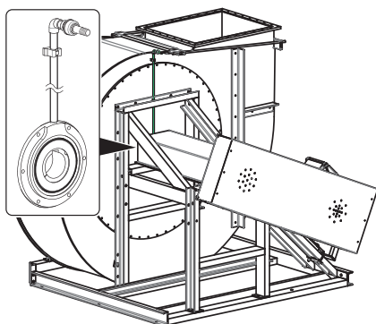
Bild 14: Spärrgasanslutning
