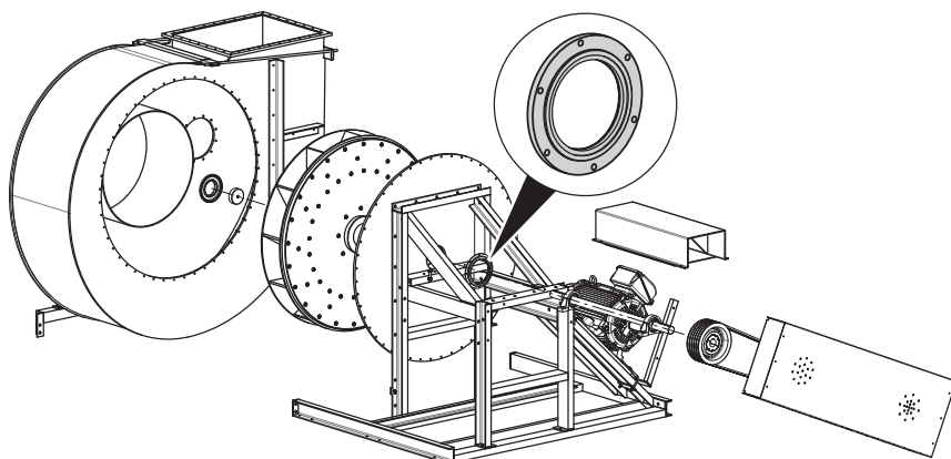
Bild 42: Ersätt läpptätning
