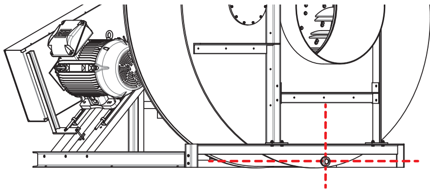
Bild 31: Kondensatstosens korrekta position
