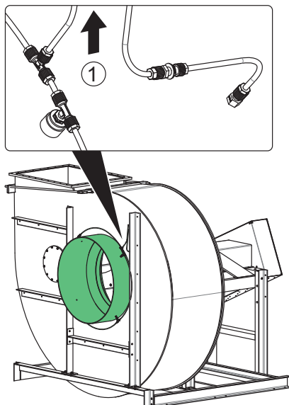
Bild 18: Mätpunkt för flödesvolym
