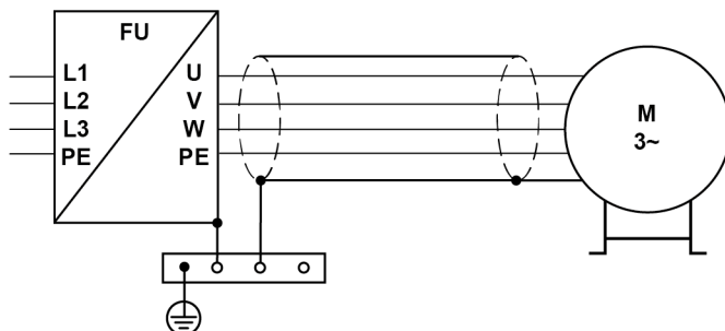
Bild 35: Anslutningsprincip för kort motorkabel (FO nära fläkten)
