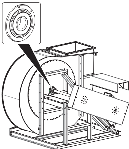
Bild 11: Läpptätning (enkel)
