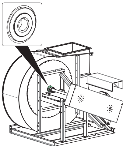
Bild 15: Filtring navtätning
