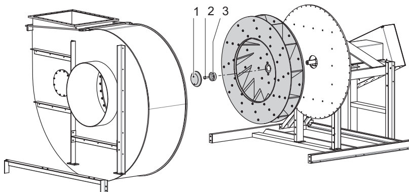
Bild 39: Byta fläkthjul
