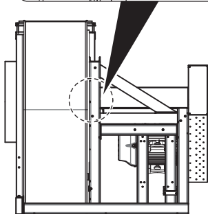
Bild 16: Labyrint-navtätning
