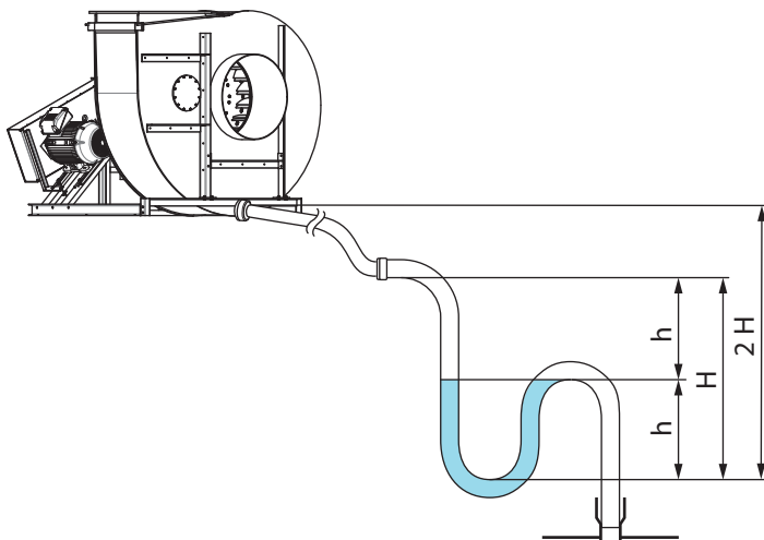
Bild 32: Sifon- och monteringshöjd
