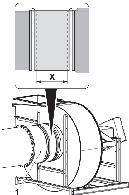
Bild 30: Röranslutningarnas distansområde
