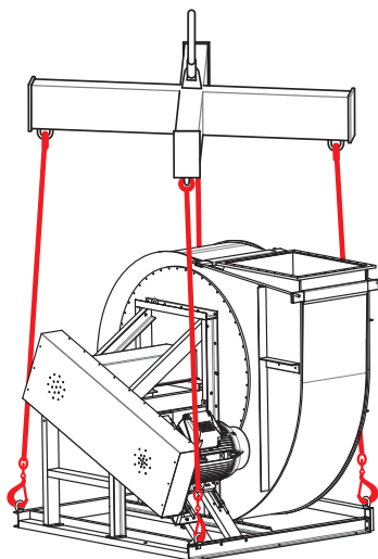
Bild 23: Fläkt på travers
