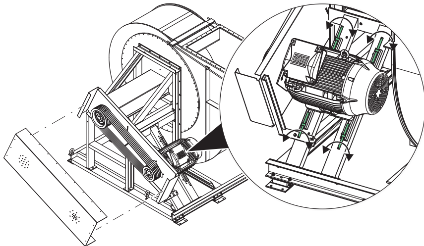
Bild 45: Ersätt drivrem
