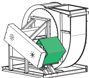
Bild 10: Motorkåpa
