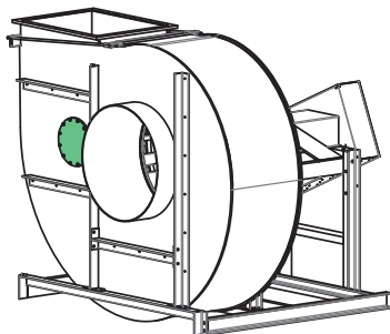
Bild 28: Korrekt montering av kontrollöppning
