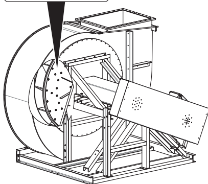
Bild 17: Fläkthjul med bakplåtar
