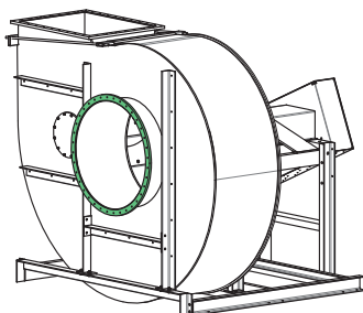
Bild 7: Rund flänsanslutning
