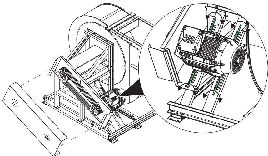
Bild 27: Kontrollera remdrift
