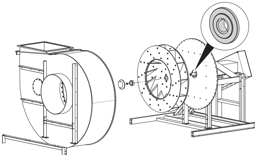
Bild 43: Ersätt filtring navtätning
