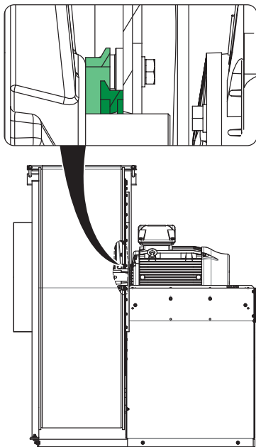
Bild 16: Labyrint-navtätning
