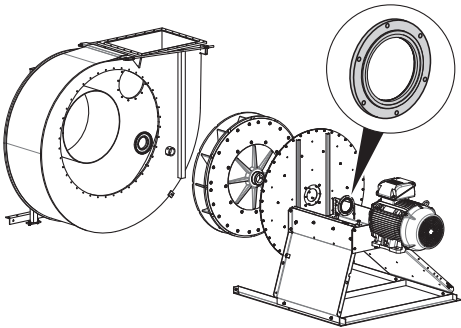
Bild 39: Ersätt läpptätning
