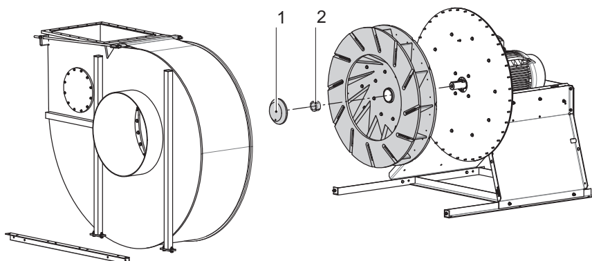
Bild 37: Byta fläkthjul
