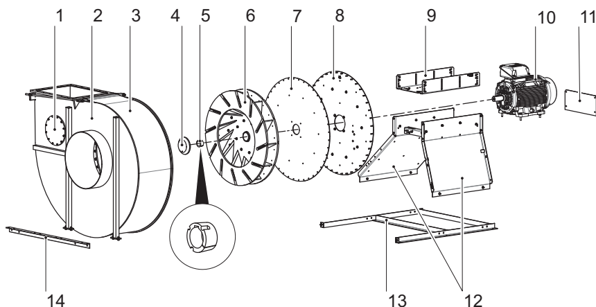
Bild 2: Fläkt-översikt
