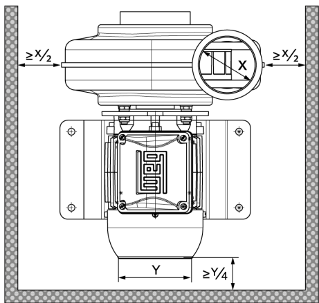
Bild 11: Platsbehov för arbetsområde och motorkylning
