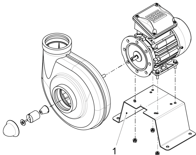
Bild 19: Demontera elmotor
