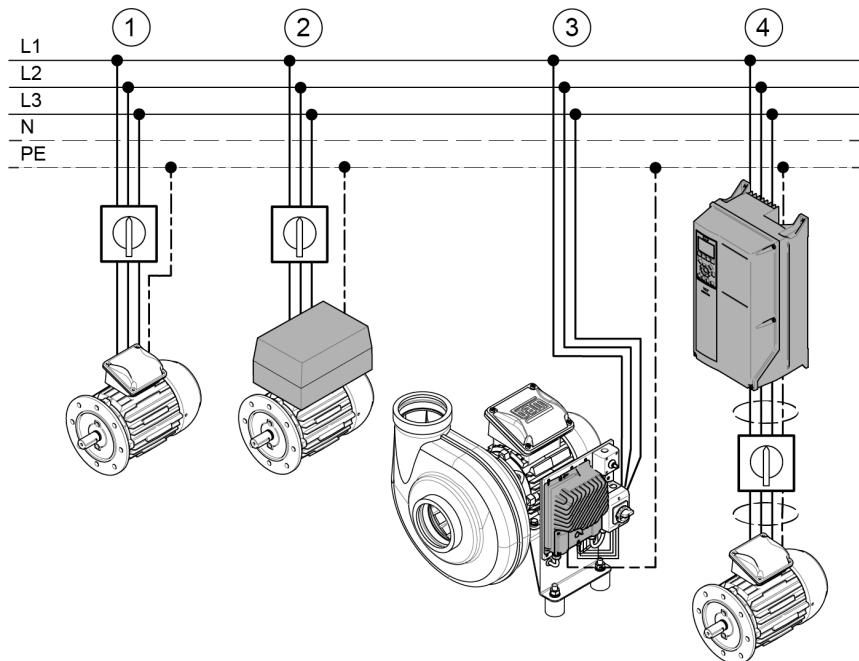
Bild 14: Frekvensomformarens (FO) monteringsmöjligheter
