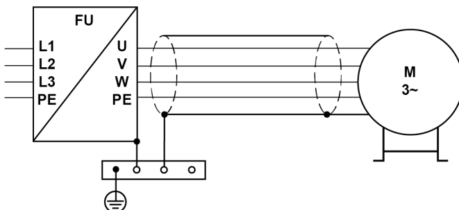
Bild 15: Anslutningsprincip för kort motorkabel (FO nära fläkten)
