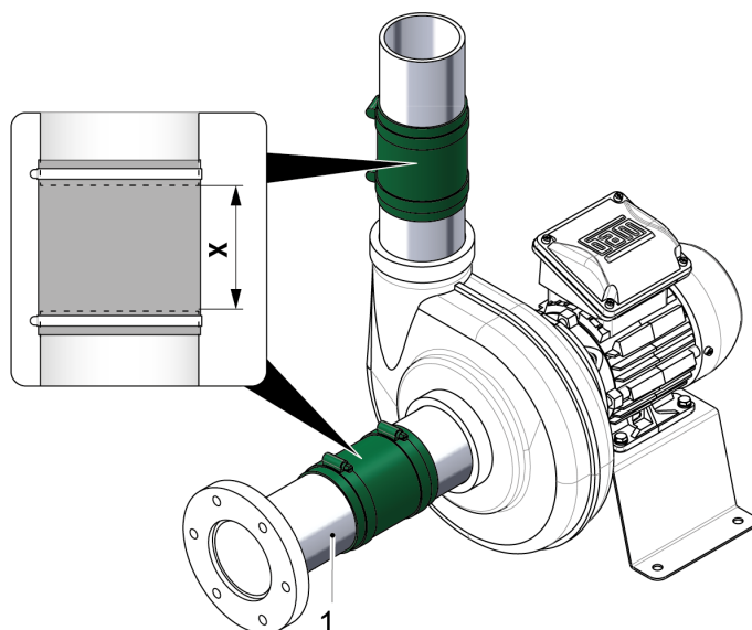
Bild 13: Röranslutningarnas distansområde
