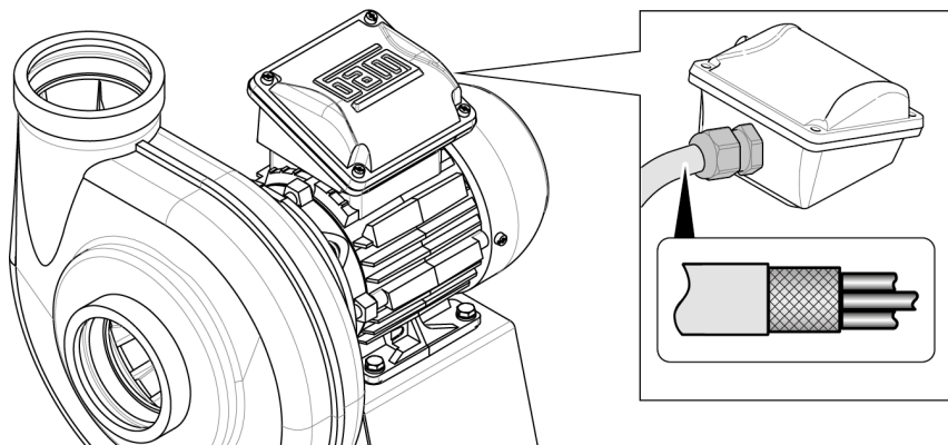
Bild 16: EMC-kabelförskruvning
