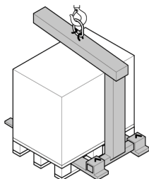
Bild 9: Kolli på transportpall
