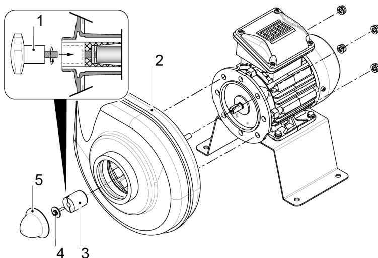
Bild 18: Demontera fläkthjul med hus
