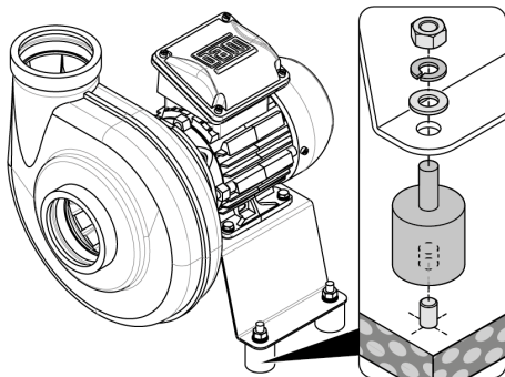
Bild 12: Fastsättningsförslag för golvmontering
